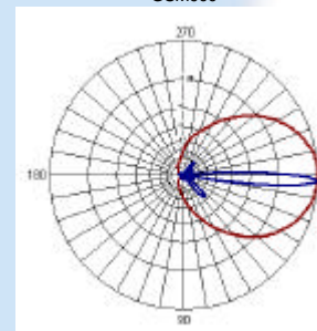
GSM 1800
