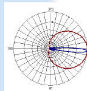
GSM900
